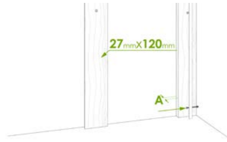
Abb. 4c: Montage Wandanschlussprofil A = Abstand von Wand zu Außenkante Unterkonstruktion
