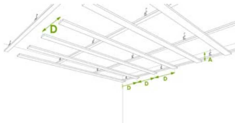
Abb. 2b Zweite Unterkonstruktion mit Holzlattung Achsabstand D=600\text{mm} (zwingend erforderlich!)
