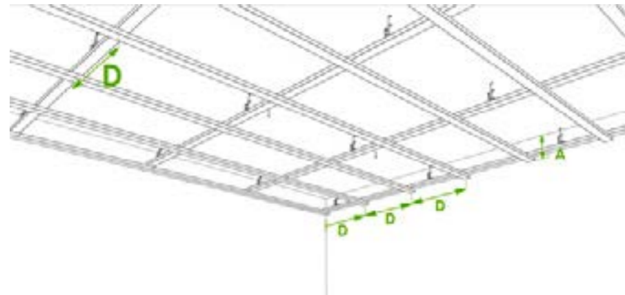
Abb. 2a Zweite Unterkonstruktion mit Stahlblechprofilen Achsabstand D=600\text{mm} (zwingend erforderlich!) A = Abstand von Rohdecke zu Unterkante der zweite Unterkonstruktion
